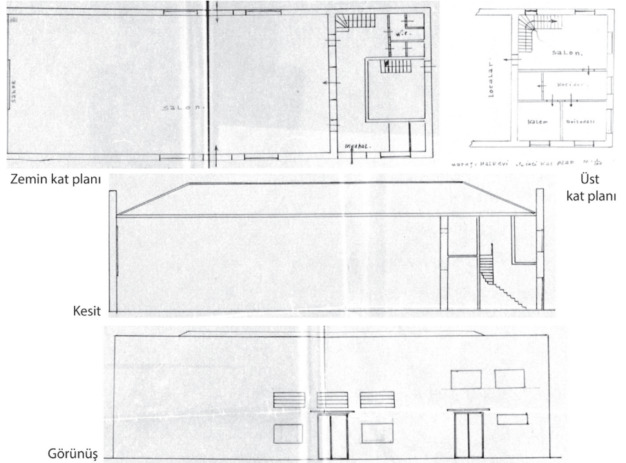
Resim 5. Maraş Halkevi için ilk tasarıya ait olduğu düşünülen kat planları, kesit ve görünüş (490-1-0-0, 1763-1156-1, 81 ve 82).
