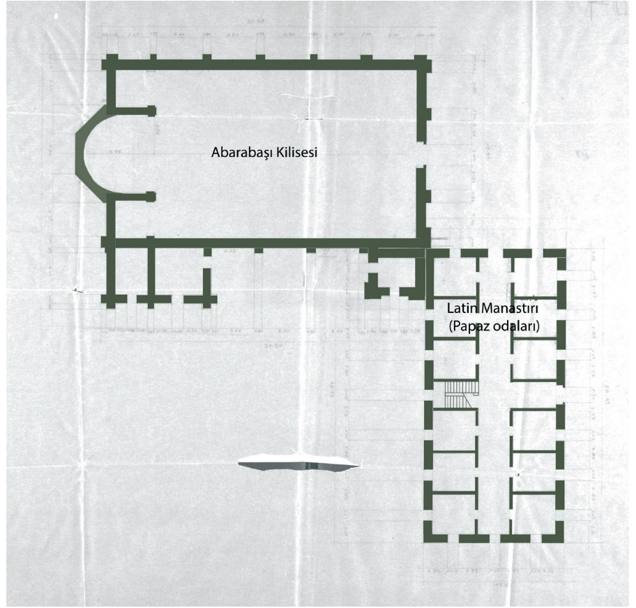
Resim 6. Halkevi arsasındaki yıkılması planlanan kilise ve yanındaki papaz odalarına ait plan (mevcut görseldeki okunaksız duvarlar, yazar tarafından koyulaştırılmıştır) (490-1-0-0, 1763-1156-1, 80).
